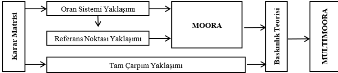
Şekil 1: MULTIMOORA Yönteminin Genel Yapısı
